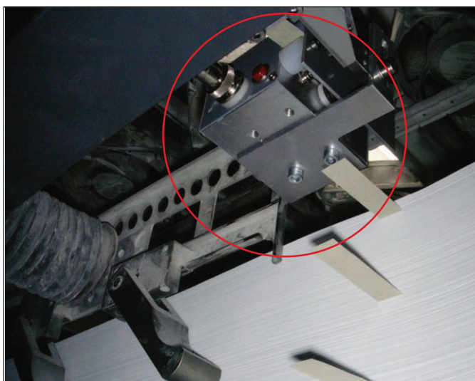
Inseritore montato su una macchina da stampa.
